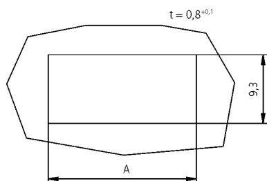
Blechausschnitt Plate cut out
